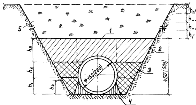
Рис. 4. Схема уплотнения грунта при засыпке траншей:
