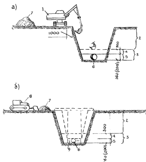
Рис. 4.2. Схема организации работ по засыпке траншей:
