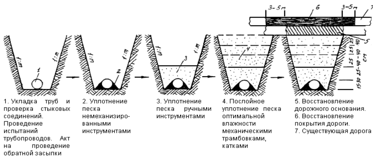
Рис.2. Последовательность работ по восстановлению дорожной конструкции
