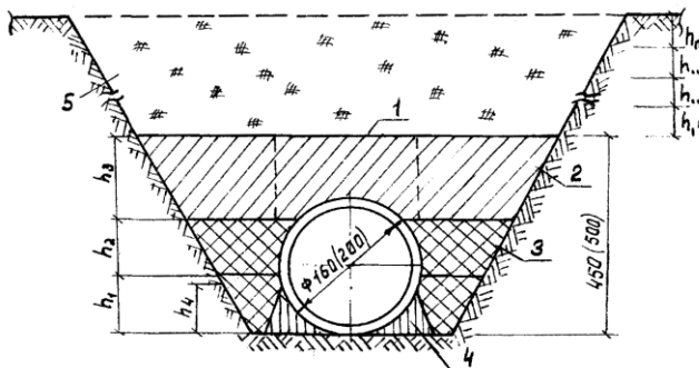
Рис. 4. Схема уплотнения грунта при засыпке траншеи:
