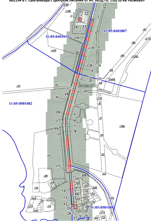
Схема расположения границ публичного сервитута объекта электросетевого хозяйства: ВЛ 10 кВ яч. 3, 10 ТП 10/0,4 кВ №378 до яч. 1 ТП 10/0,4 кВ №2194 в г. Сыктывкаре с центром питания от яч. 361Д ПС 110/10 кВ «Южная»
