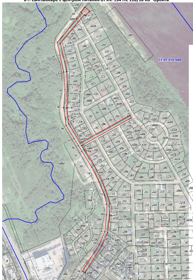
Схема расположения границ публичного сервитута объекта электросетевого хозяйства: ВЛ 10 кВ от линейного разъединителя №273 через КТП №№1138, 1137, 1136, 1132, 1127, 1126, 1125 до КТП 10/0,4 кВ №1124 по проезду Геологов в г. Сыктывкаре с центром питания от яч. 934 ПС 110/10 кВ "Орбита"
