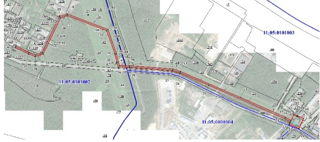
Схема расположения границ публичного сервитута объекта электросетевого хозяйства: ВЛ-10кВ ПС"ЧОВЬЮ" ф.426-РП-11 ф.24
