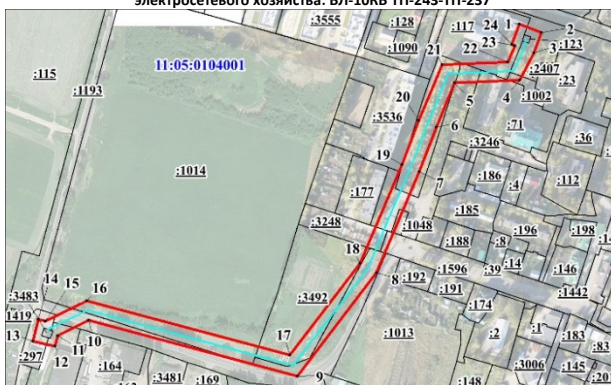
Схема расположения границ публичного сервитута объекта электросетевого хозяйства: ВЛ-10кВ ТП-243-ТП-237
