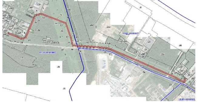
Схема расположения границ публичного сервитута объекта электросетевого хозяйства: ВЛ-10кВ ПС"ЧОВЬЮ" ф.421-РП-11 ф.19
