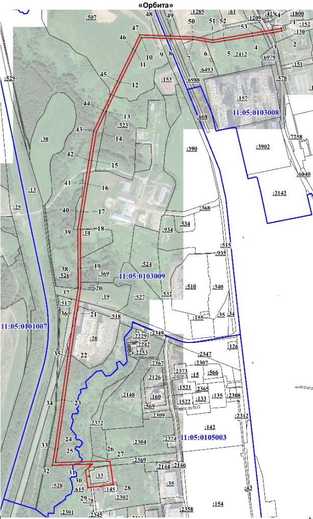
Схема расположения границ публичного сервитута объекта электросетевого хозяйства: ВЛ 10кВ от яч. 942, 953 ПС 110/10 кв «Орбита» до яч. 8, 19 РП 10/0,4 кв №8 в г. Сыктывкаре с центром питания от яч. 942, 953 ПС 110/10 кв «Орбита»
