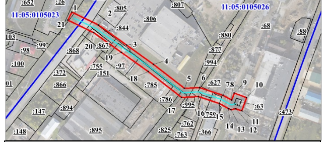
Схема расположения границ публичного сервитута объекта электросетевого хозяйства: ВЛ-10кВ ТП-231-ТП-226 Л-1
